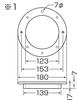
※1 固定板寸法図
