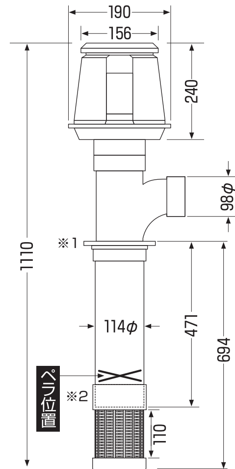
※2 ストレーナー寸法図
