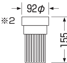
※1 ※2 82 固定板寸法図 83 ストレーナー寸法図
