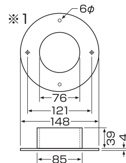
※1 固定板寸法図
