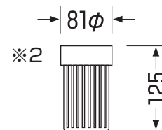
※2 ストレーナー寸法図
