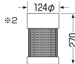
※2 ストレーナー寸法図
