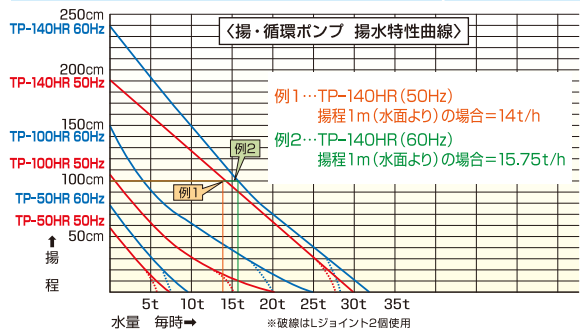
TP-50HR TP-100HR TP-140HR TP-30R 揚・循環ポンプ 循環のみ
