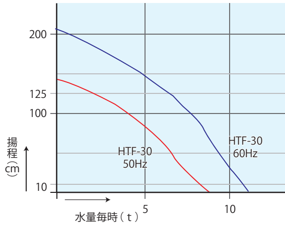
HTF 型汲み揚げポンプ特性曲線
